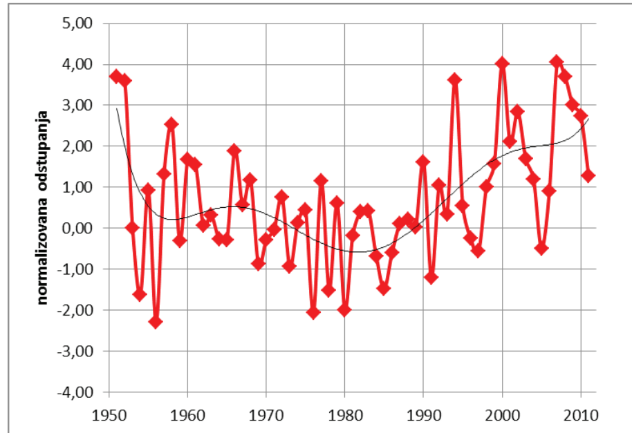
Grafikon 1. Temperaturni uslovi za region Pomoravlja: period 1951-2011.
