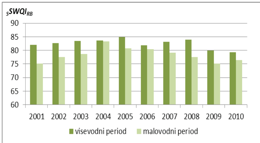
Grafik 2: Vrednosti sezonskog indikatora kvaliteta vode sliva Zapadne Morave
