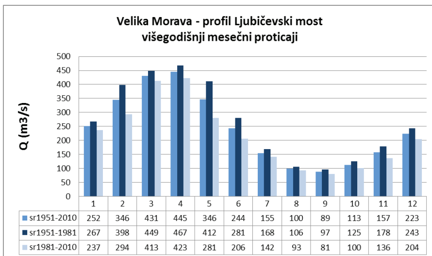
Grafikon 3: Višegodišnji srednji mesečni proticaji reke Velike Morave na profilu Ljubičevski most
