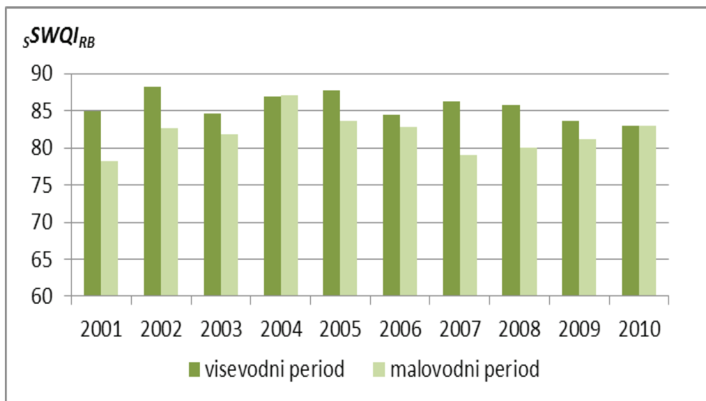
Grafik 1: Vrednosti sezonskog indikatora kvaliteta vode sliva Južne Morave
