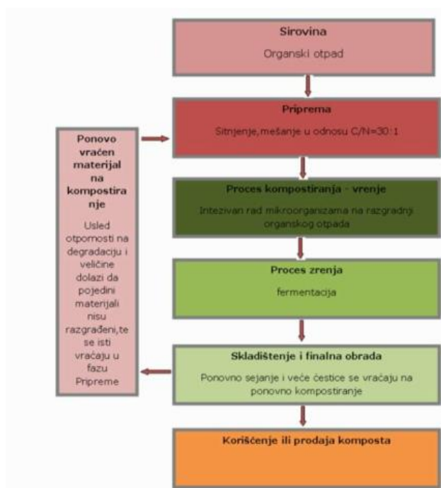
Слика 14. Приказ фаза технолошког процеса компостирања
