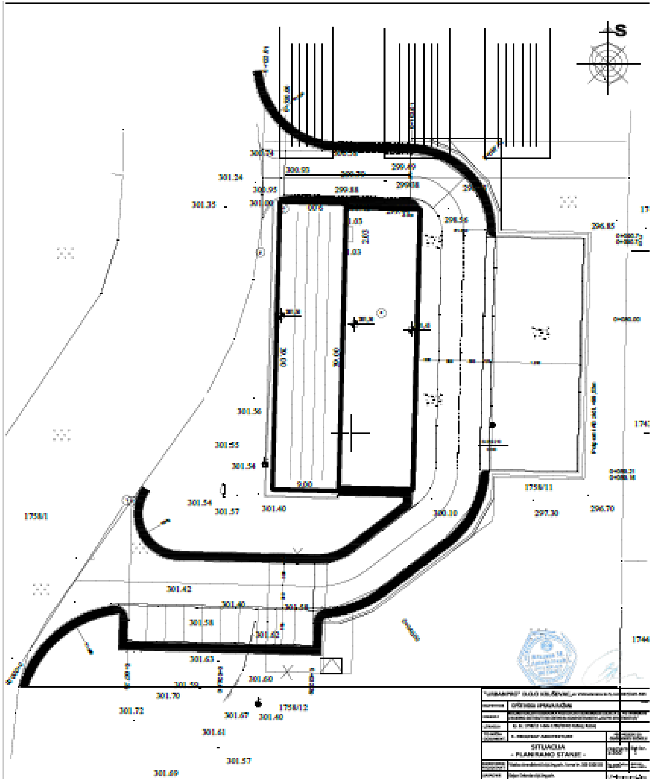
Слика 30. Ситуациони план рециклажног центра
