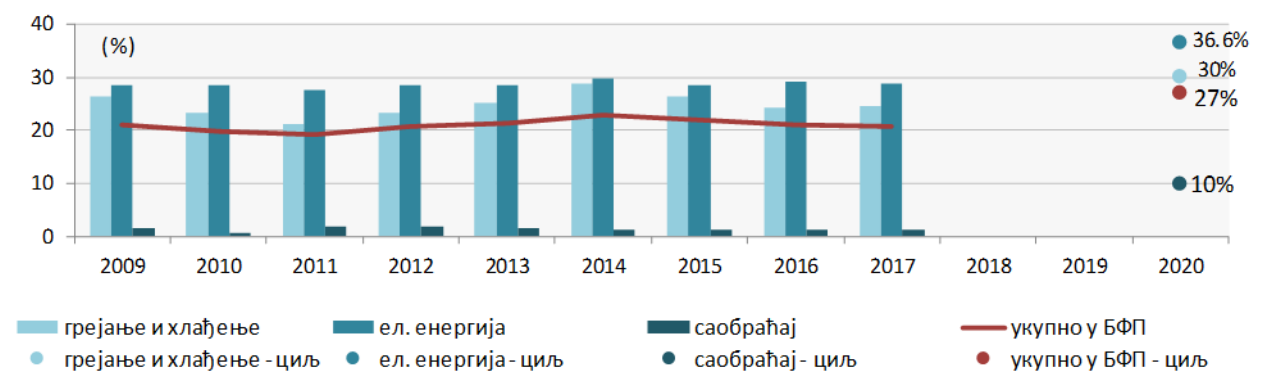
Слика 160. Учешће ОИЕ у потрошњи енергије по секторима и у бруто финалној потрошњи енергије (БФПЕ)
