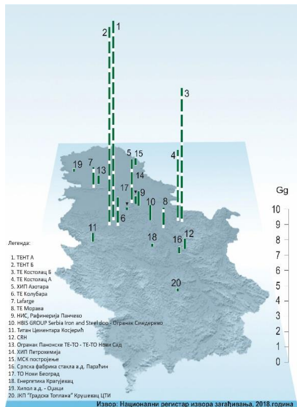
Слика 2. Емисије оксида азота из 20 највећих извора у Републици Србији (Gg) у 2018. години
