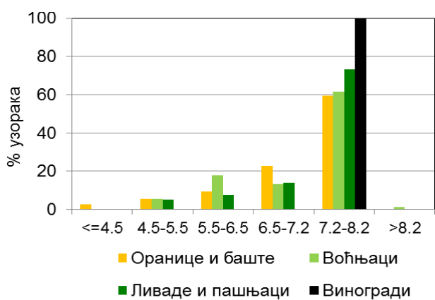
Слика 90. Супституционална киселост (pH у nKCl-у)
