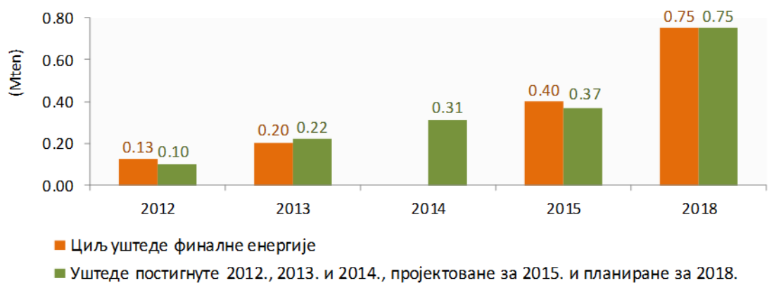
Слика 157. Преглед циљева и остварених/планираних уштеда финалне енергије (Mten)
