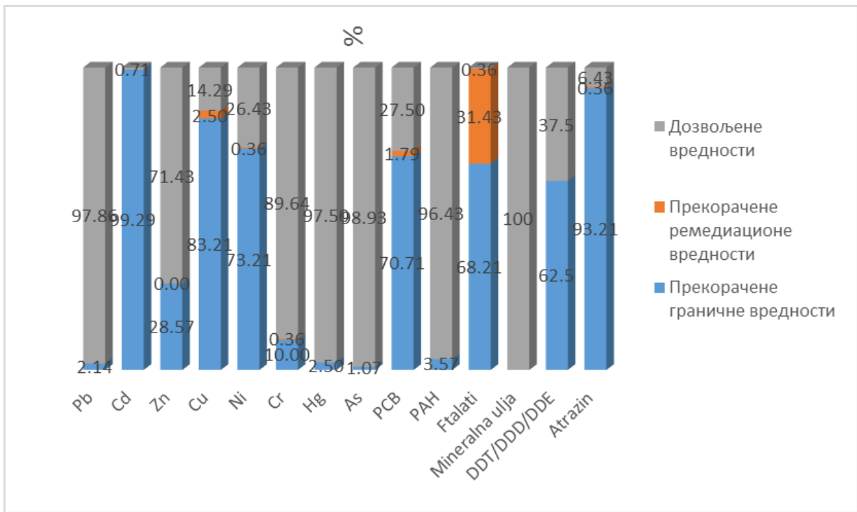
Слика 101. Процент прекорачења испитиваних параметара на дубини од 30-60 cm
