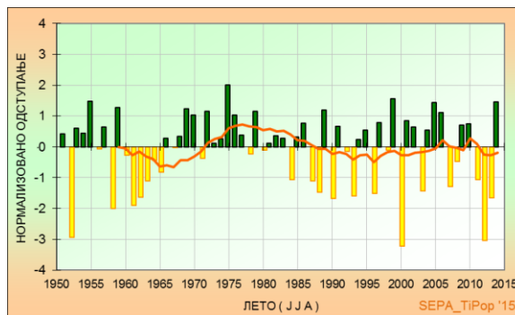
Слика 28. Нормализована одступања, са десетогодишњим клизним средњаком, годишњих (лево) и летњих (десно) количина падавина у Републици Србији, период 1951-2014. година.
