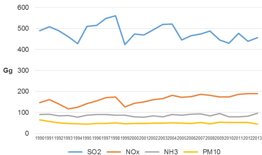
Слика 12. Емитоване количине примарних суспендованих честица и секундарних прекурсора суспендованих честица у Републици Србији у периоду 1990-2013
