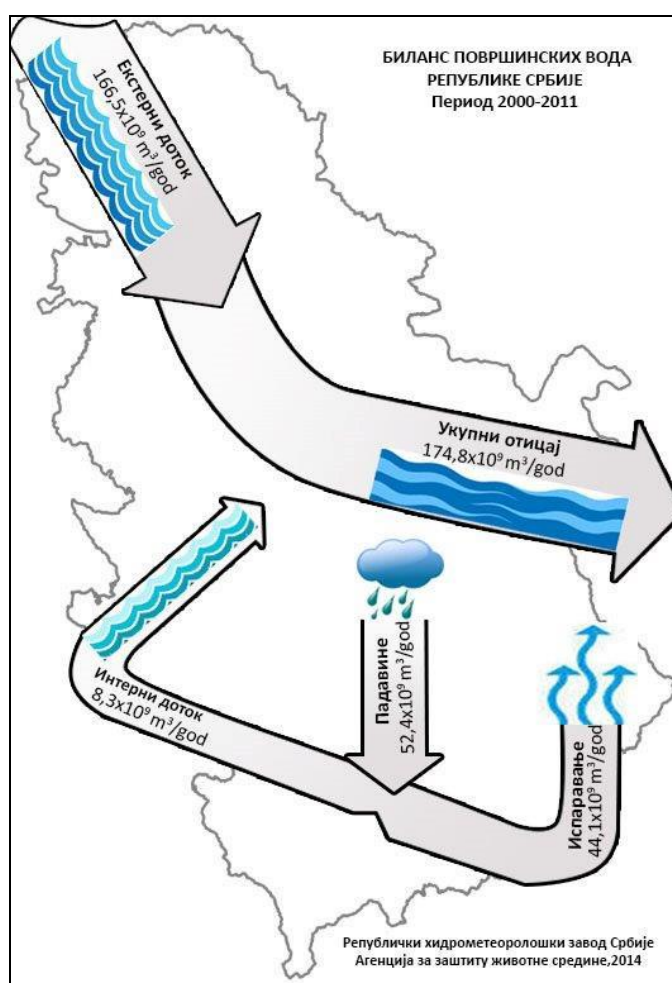
Слика 116. Обновљиви водни ресурси Србије у периоду 2000-2011. година
