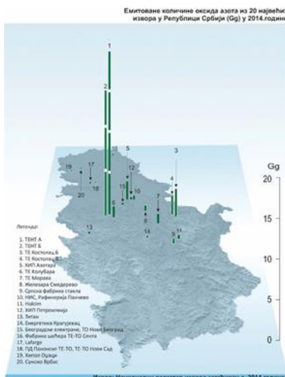
Слика 3. Емисије оксида азота
