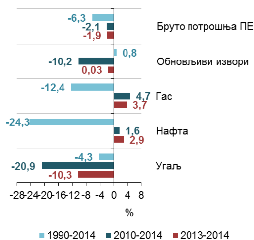
Слика 143. Стопе раста потрошње различитих енергената у %.
