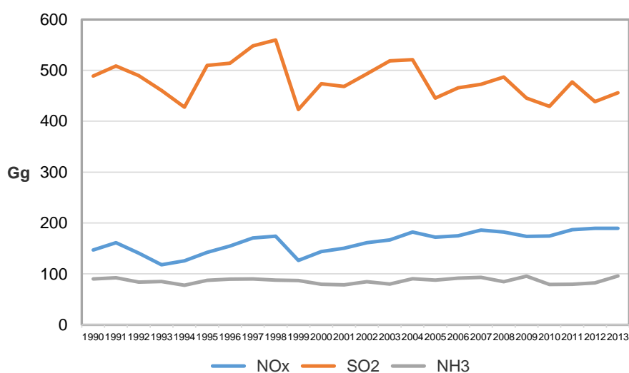
Слика 5. Тренд емисија закисељавајућих гасова од 1990. до 2013. (Гг/год)
