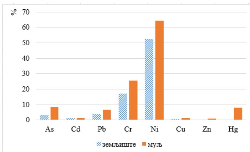
Слика 190. Процент прекорачења МДК у узорцима земљишта и муља на поплављеном подручју
