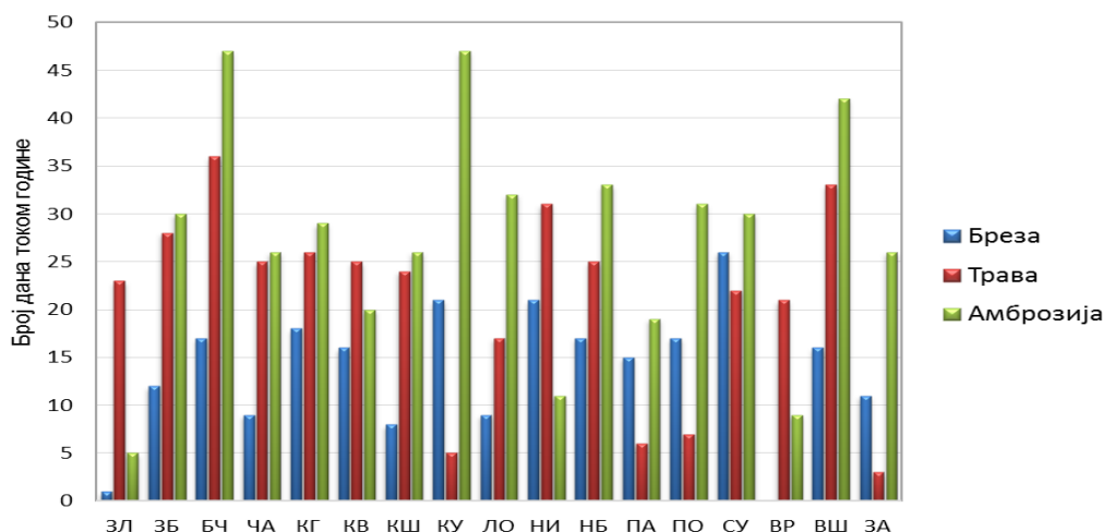
Слика 24. Број дана са прекорачењем граничних вредности алергеног полена у мрежи станица за 2014. годину
