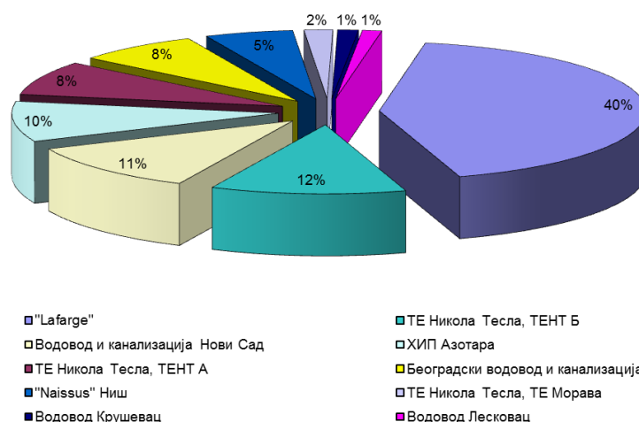
Слика 56. Удео у укупној емисији азота у отпадним водама из тачкастих извора – 10 највећих извора загађивања у Републици Србији у 2014. години
