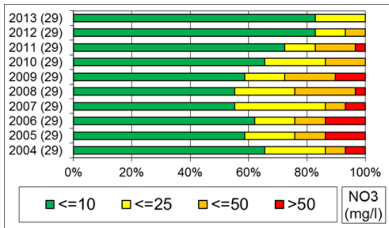
Слика 50. Расподела учесталости нитрата у подземним водама Србије (2004-2013.)
