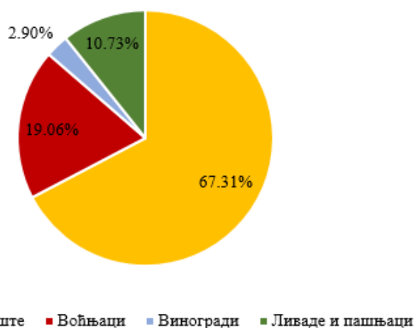
Слика 68. Процентуални удео узорка према начину коришћења земљишта
