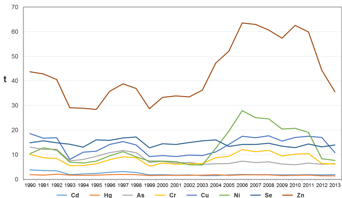
Слика 14. Емитоване количине Hg, Cd, As, Cu, Cr, Ni, Se, Zn у Републици Србији у периоду 1990-2013. година
