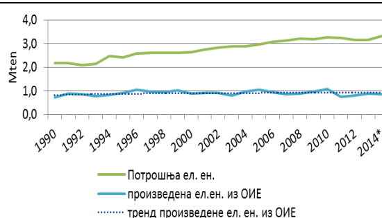
Слика 152. Потрошња електричне енергије и произведена ел. ен. из ОИЕ
