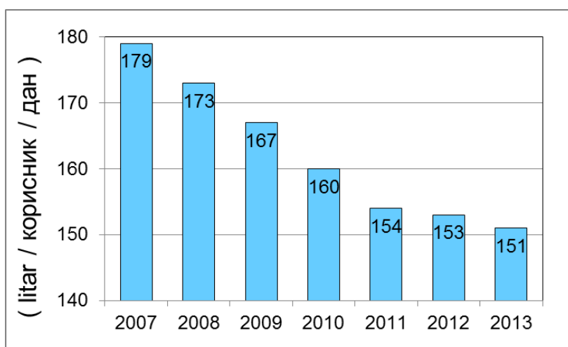
Слика 120. Коришћење воде у домаћинству
