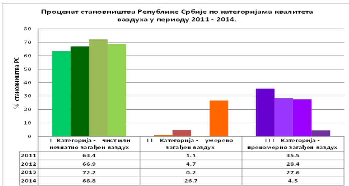
Слика 23. Процент становништва Републике Србије изложен различитом степену загађења у зависности од оцене квалитета ваздуха
