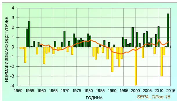
Слика 28. Нормализована одступања, са десетогодишњим клизним средњаком, годишњих (лево) и летњих (десно) количина падавина у Републици Србији, период 1951-2014. година.
