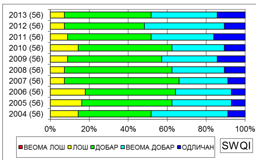
Слика 46. Расподела учесталости SWQI у водотоцима Републике Србије (2004-2013.)
